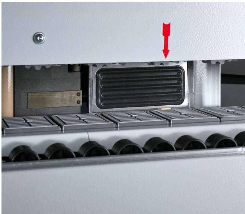
Halogenový zářič pro ohřev dílců
